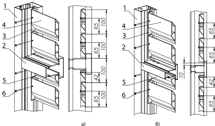
Рис. 31. Заполнение алюминиевым профилем «жалюзи» при наличии горизонтального импоста:
