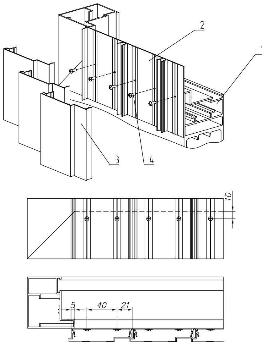
Рис. 26. Накладной тип монтажа сплошного заполнения:
