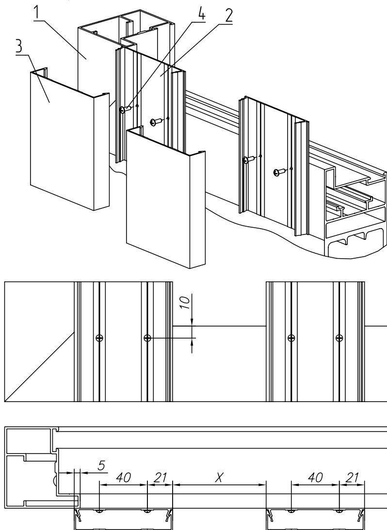
Рис. 21. Накладной тип монтажа разреженного заполнения профилем 82 мм:
