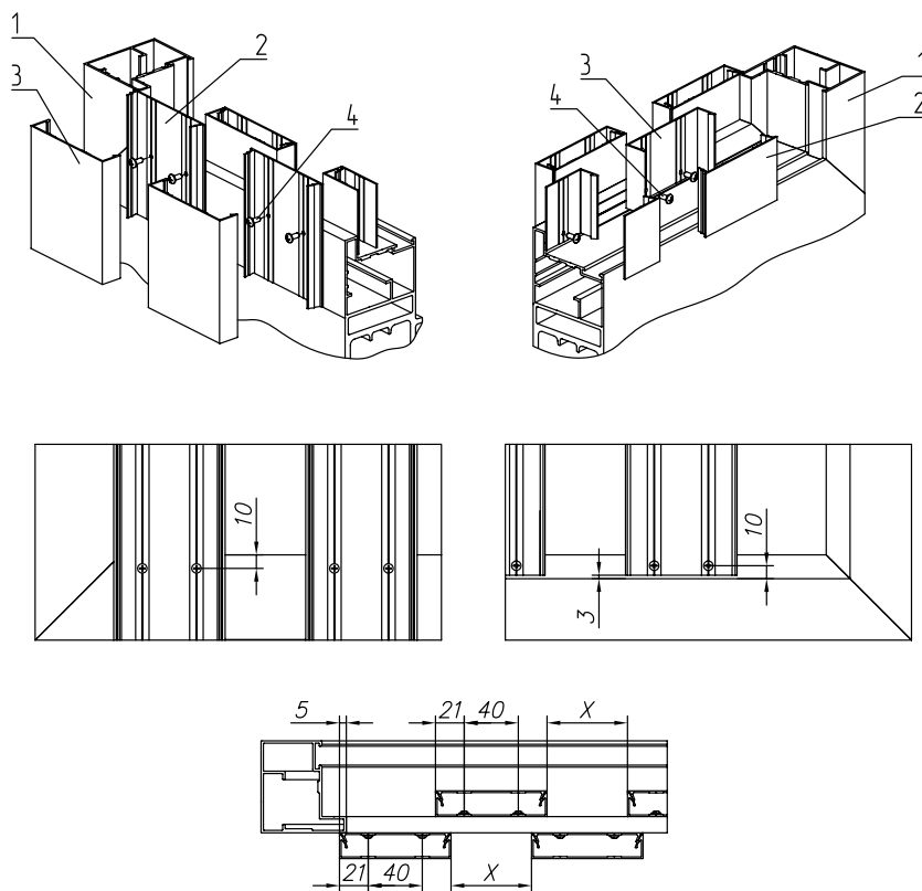
Рис. 24а. Шахматное заполнение профилями шириной 82 мм:
