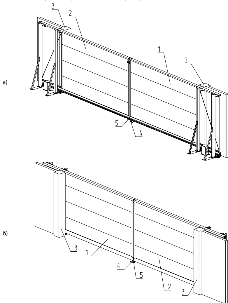
Рис. 70. Встречные откатные самонесущие ворота:
