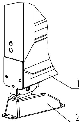
Рис. 72. Установка упора FLGU.400.0933 (для ворот на профиле 68 мм), FLGU.400.0948 (для ворот на профиле 96 мм)
