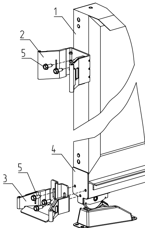
Рис. 73. Установка верхнего и нижнего улавливателей
