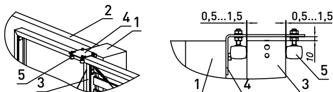
Рис. 53. Установка кронштейна SGN.02.717 в откатных самонесущих воротах при монтаже ворот без столба удерживающего:
