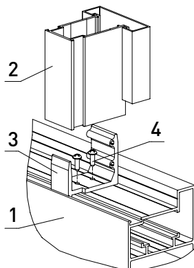
Рис. 4. Установка вертикального импоста:
