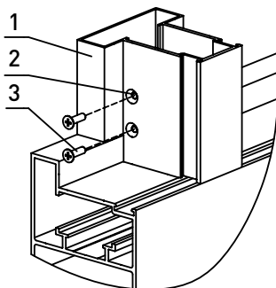
Рис. 8. Крепление импоста:
