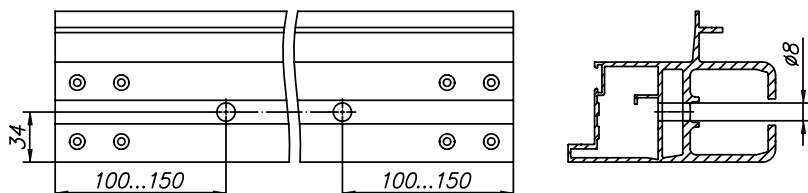
Рис. 10б. Изготовление дренажных отверстий
