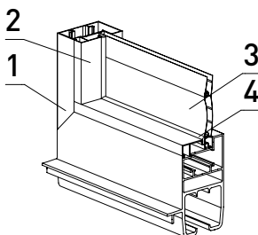
Рис. 37. Установка штапика с уплотнителем FRK39 :
