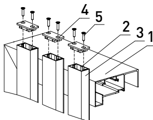
Рис. 28. Установка крышек FLGU.400.0703 :
