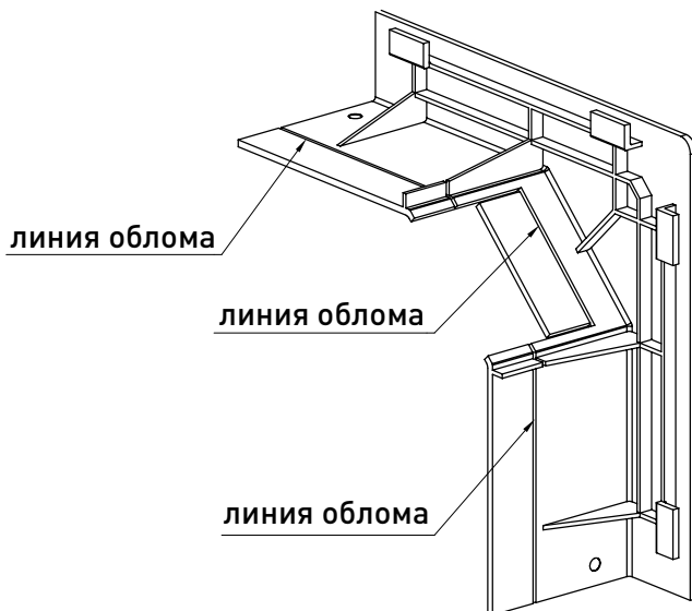
Рис. 41. Крышка FLGU.400.0717
