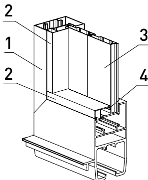
Рис. 38. Установка штапиков с уплотнителем FRK12 :
