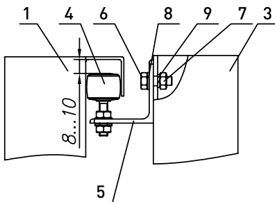
Рис. 50. Установка столба удерживающего:
