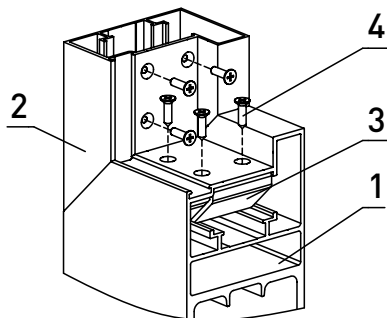
Рис. 10а. Крепление углов:
