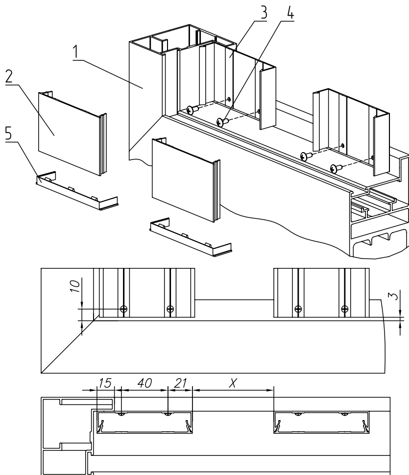
Рис. 18. Встроенный тип монтажа разреженного заполнения профилем 82 мм:
