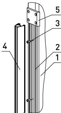
Рис. 47. Установка демпфирующего элемента:
