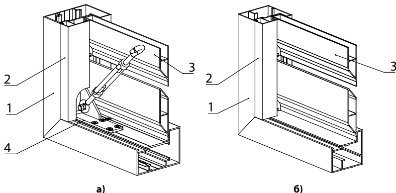
Рис. 39. Установка штапиков в раму с заполнением «жалюзи»
