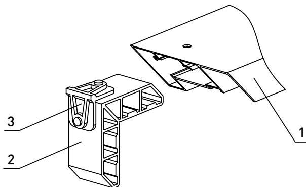
Рис. 6. Установка соединителей угловых в балку:
