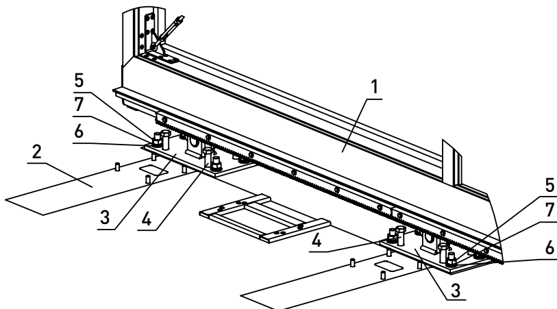
Рис. 49. Установка створки ворот на раму опорную:
