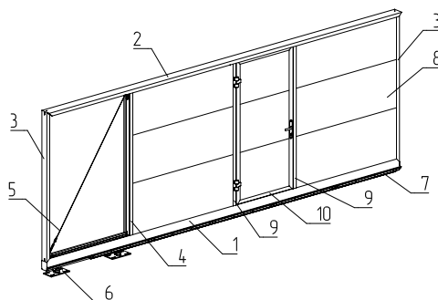
Рис. 64. Откатные ворота со встроенной калиткой
