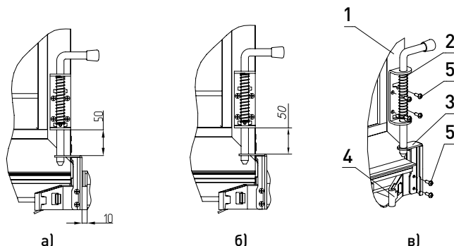
Рис. 63. Установка засова с применением кронштейна FLGU.400.0939 ( FLGU.400.0940 )
