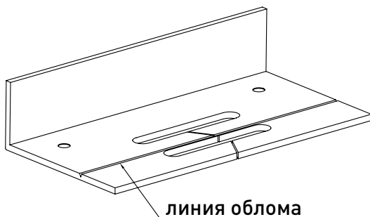
Рис. 43. Крышка FLGU.400.0723
