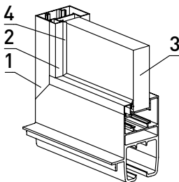
Рис. 36. Установка штапика и уплотнителя FRK12 в створку ворот:
