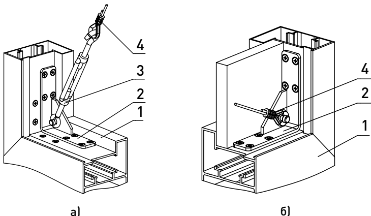
Рис. 35. Установка тросовой растяжки с талрепом:
