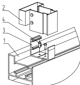
Рис. 65. Установка соединителей под вертикальный разделительный импост (столб)
