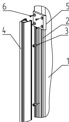
Рис. 74. Установка элементов безопасности на створку ворот:
