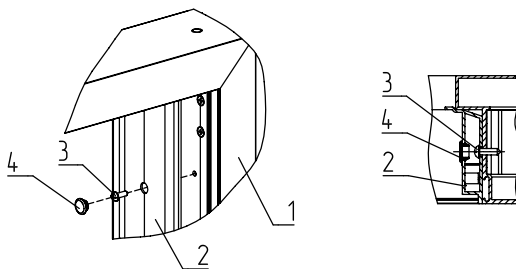
Рис. 67. Установка профиля притвора FLGU.400.0505
