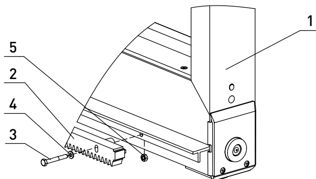
Рис. 48. Установка рейки зубчатой:
