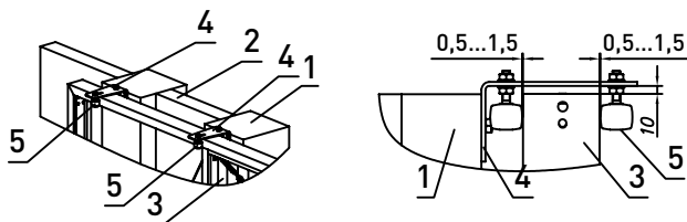
Рис. 54. Установка кронштейна FLGU.400.0918 в откатных самонесущих воротах при монтаже ворот без столба удерживающего:
