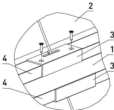
Рис. 42. Установка крышки FLGU.400.0723 :
