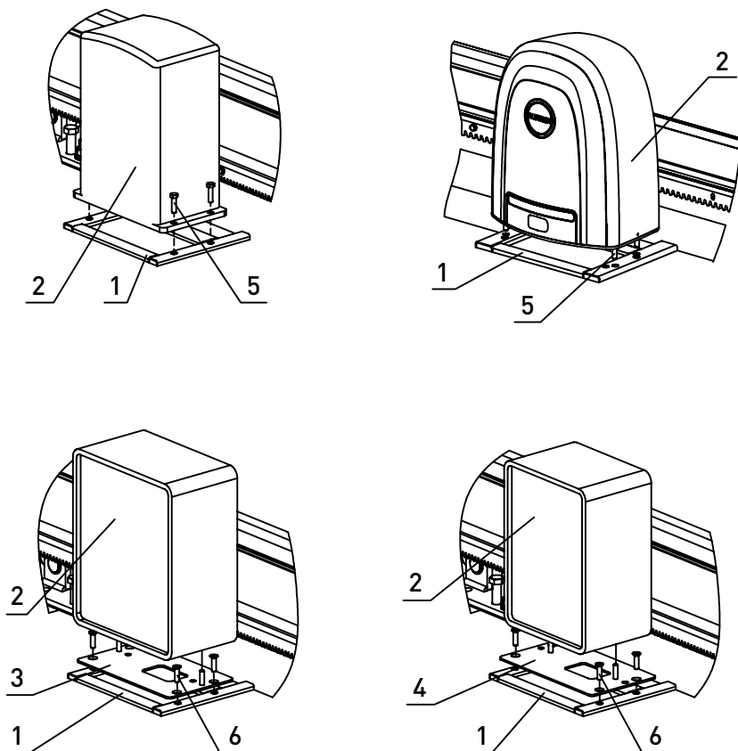
Рис. 61. Установка пластины для крепления электропривода:
