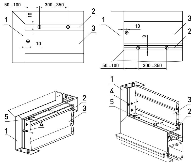
Рис. 17. Установка заполнения:
