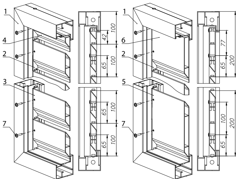
Рис. 30. Заполнение алюминиевым профилем жалюзи:
