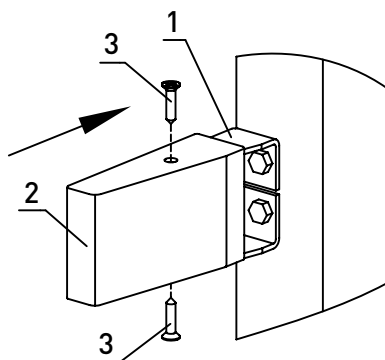
Рис. 57. Установка крышки FLGU.400.0722
