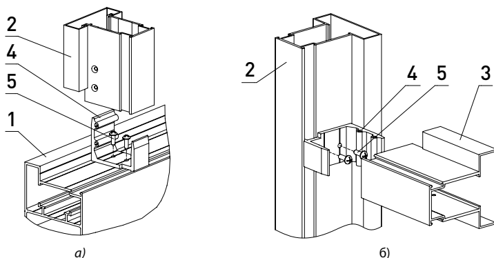
Рис. 5. Установка импостов:
