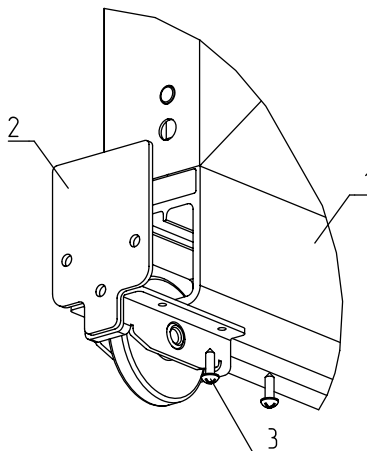
Рис. 71. Установка ролика опорного FLGU.400.0630 (для ворот на профиле 68 мм), FLGU.400.0631 (для ворот на профиле 96 мм)
