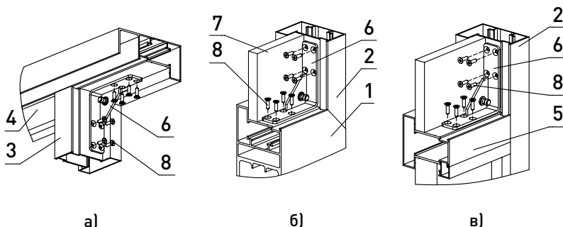
Рис. 34. Установка кронштейна FLGU.400.0906 :
