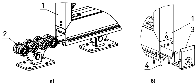
Рис. 45. Установка опор роликовых и ролика опорного:
