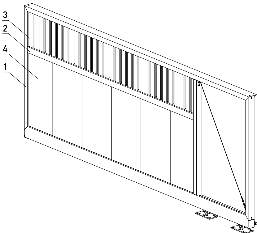
Рис. 32. Створка с комбинированным заполнением:
