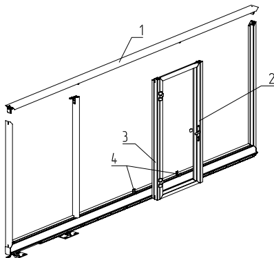
Рис. 66. Установка рамы калитки в створку распашных ворот:
