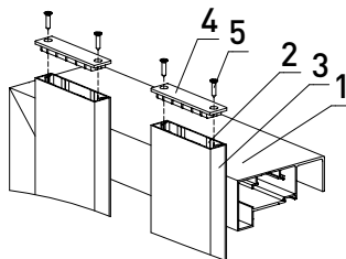
Рис. 27. Установка крышек FLGU.400.0702:
