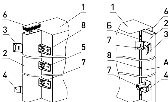
Рис. 56. Установка элементов притвора с использованием столба притвора:
