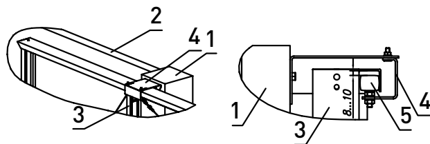
Рис. 55. Установка кронштейна FLGU.400.0919 в откатных самонесущих воротах при монтаже ворот без столба удерживающего:
