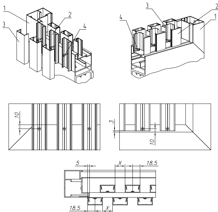
Рис. 246. Шахматное заполнение профилями шириной 37 мм:
