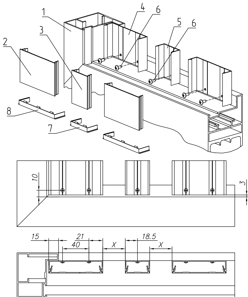
Рис. 20. Встроенный тип монтажа разреженного заполнения комбинацией профилей 82 и 37 мм:
