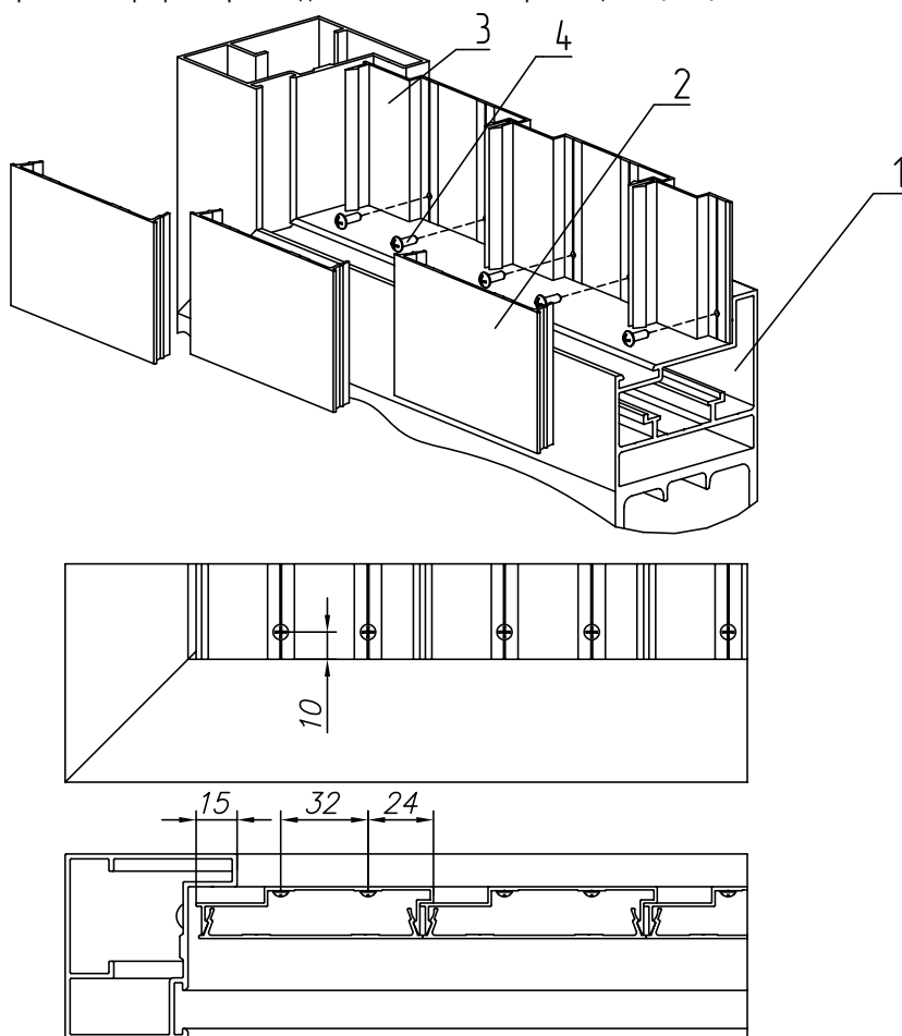
Рис. 25. Встроенный тип монтажа сплошного заполнения:
