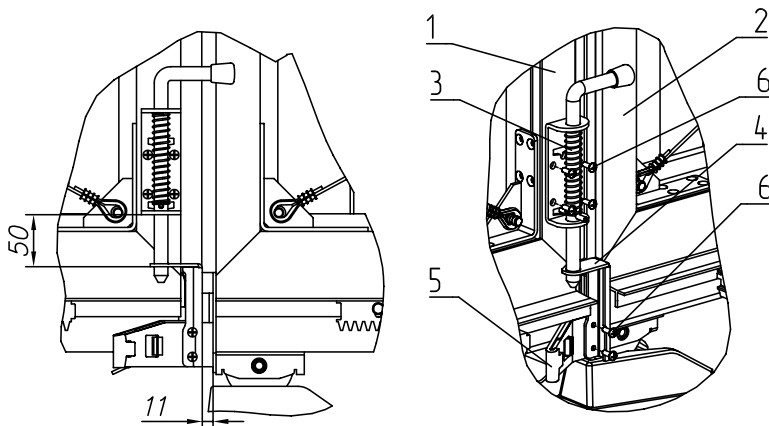
Рис. 75. Установка засова встречных откатных ворот
