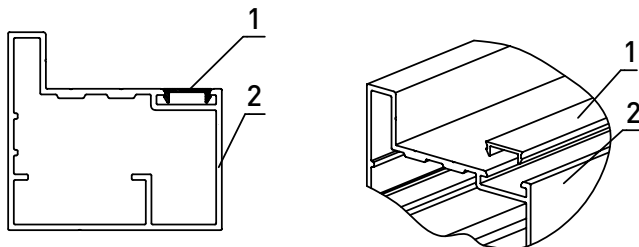
Рис. 33. Установка уплотнителя FLGU.400.0718
