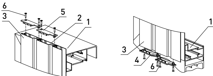
Рис. 29. Установка крышек сплошного заполнения:
