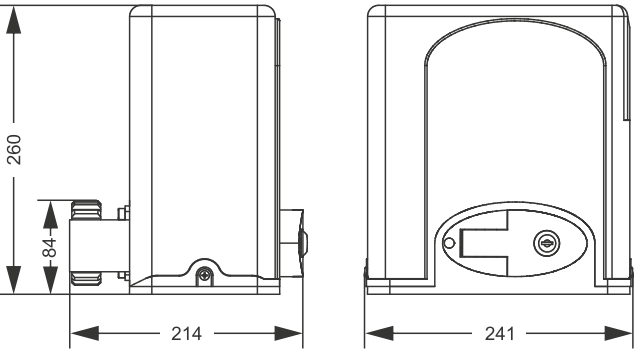
Рис. 1. Габаритные размеры привода, мм
