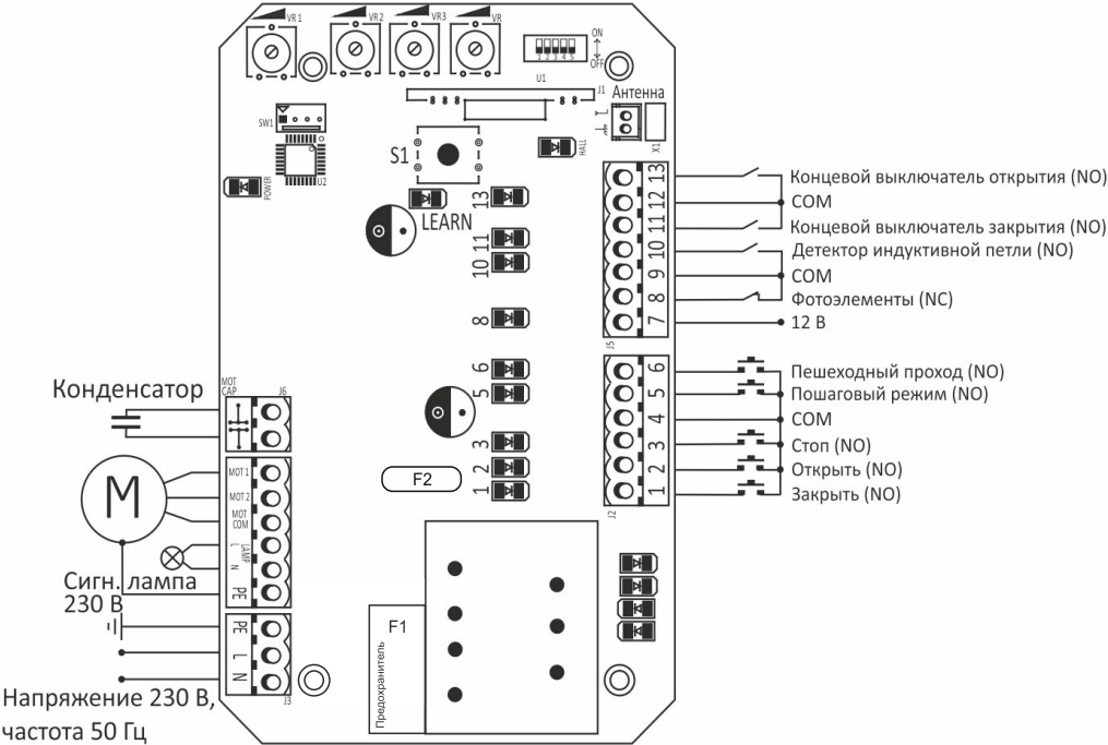
Рис. 14. Схема электрических подключений с магнитными концевыми выключателями
