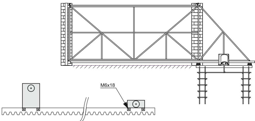
Рис. 12. Схема установки магнитов и кронштейнов магнитных концевых выключателей при установке привода справа
