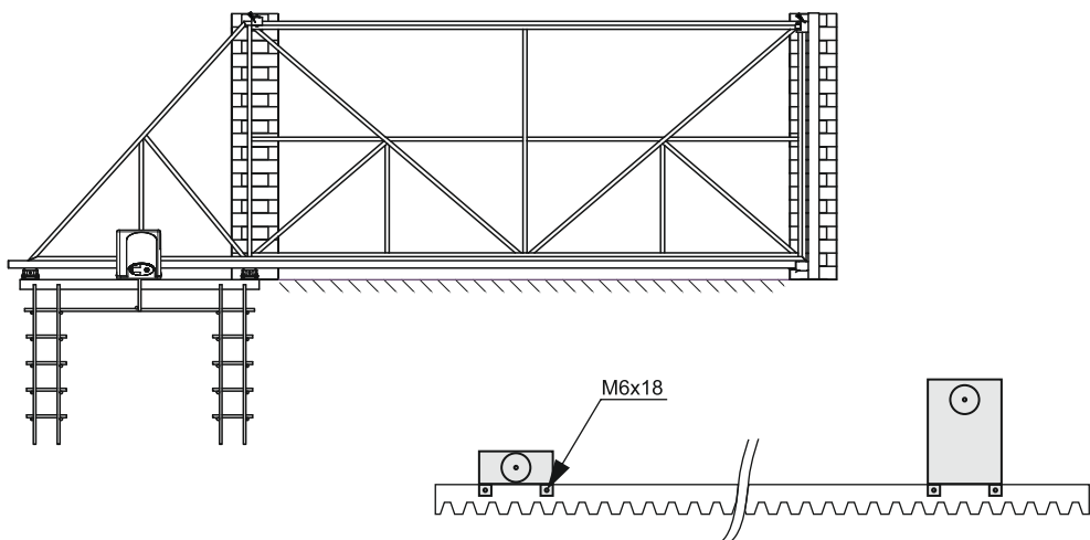
Рис. 11. Схема установки магнитов и кронштейнов магнитных концевых выключателей при установке привода слева
