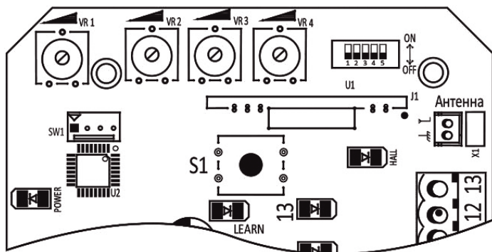
Рис. 15. Схема регулировок
