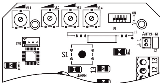
Рис. 20. Плата управления
