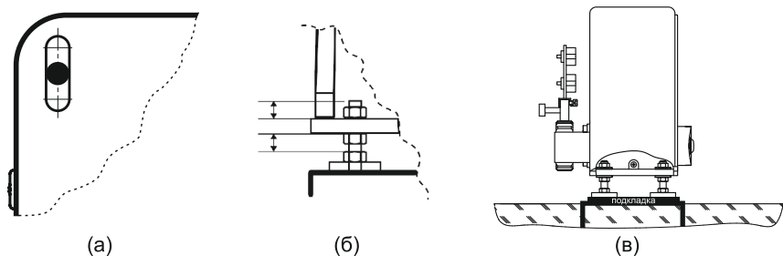
Рис. 9. Установка привода на подставку, которая идет в комплекте
