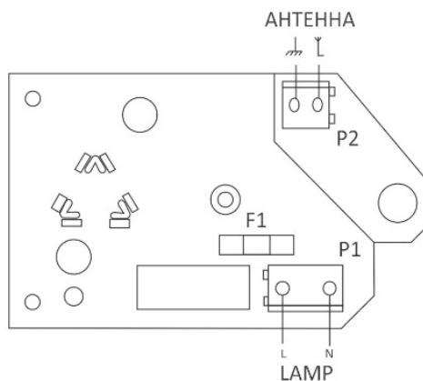
Рис. 18. Схема подключения сигнальной лампы RT-LA230V
