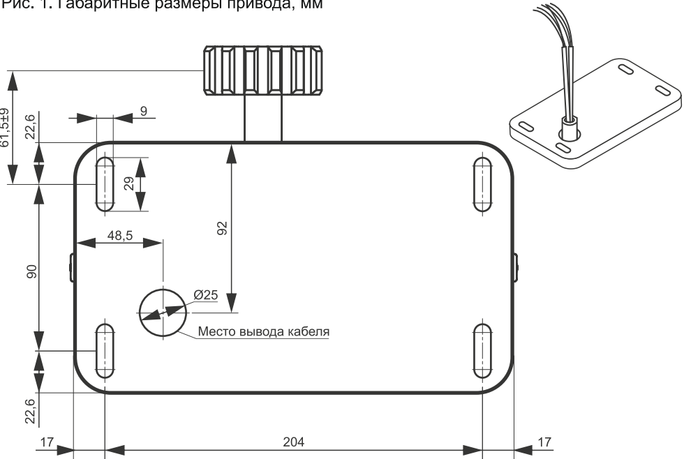
Рис. 2. Размеры для монтажа, мм (вид сверху)
