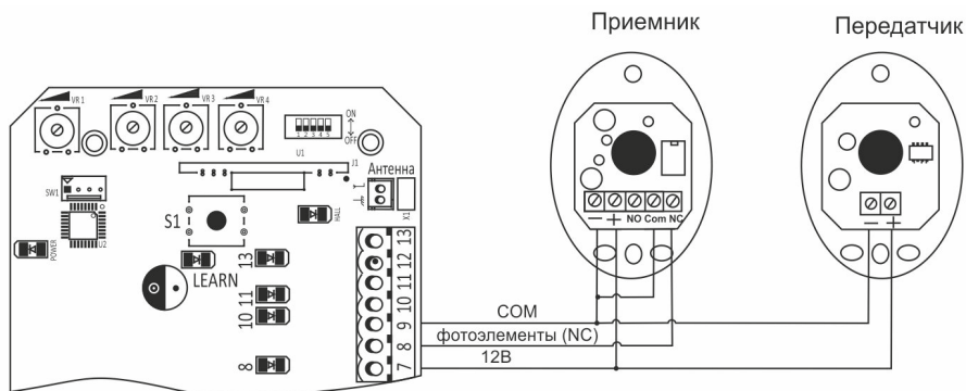
Рис. 17. Схема подключения фотоэлементов RT-F1
