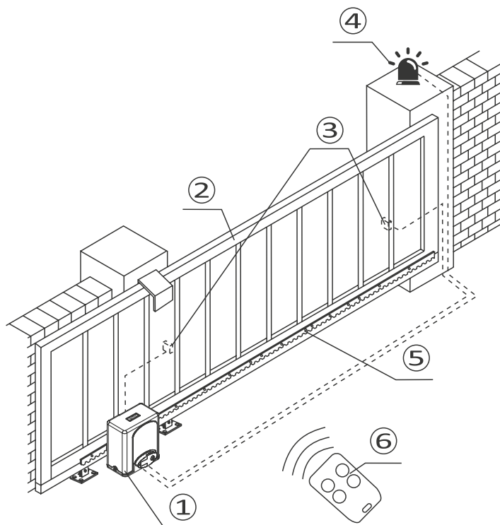
Рис. 3. Схема ворот
