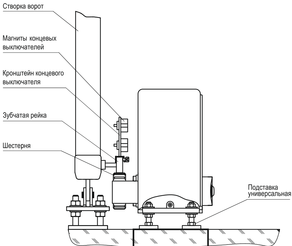
Рис. 10. Схема установки привода с магнитными концевыми выключателями
