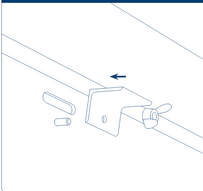
Рис. 7.14. Вид А на рис. 2
